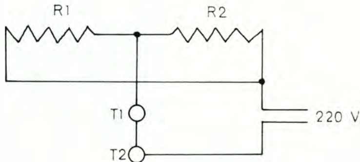
Σχ. 2 Ἡλεκτρικὸ διάγραμμα τῆς συσκευῆς συντηρήσεως.
