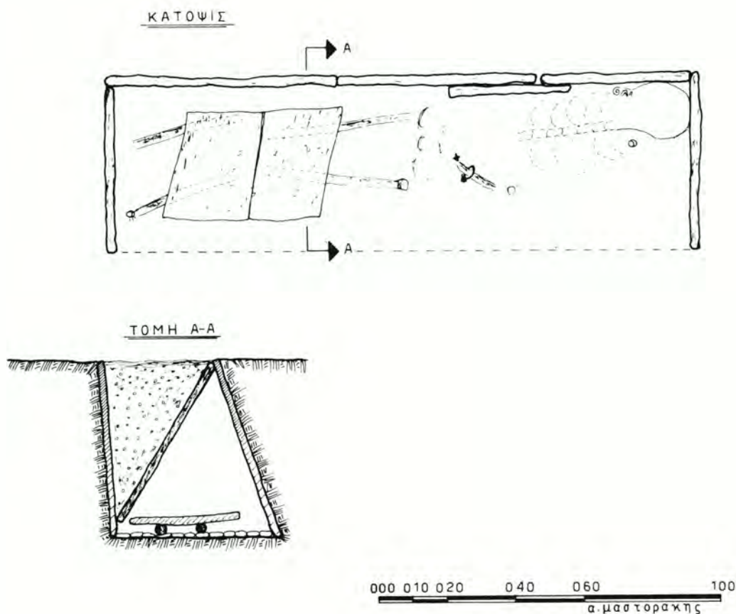
Σχ. 1. Κάτοψη και τομή τάφου.
