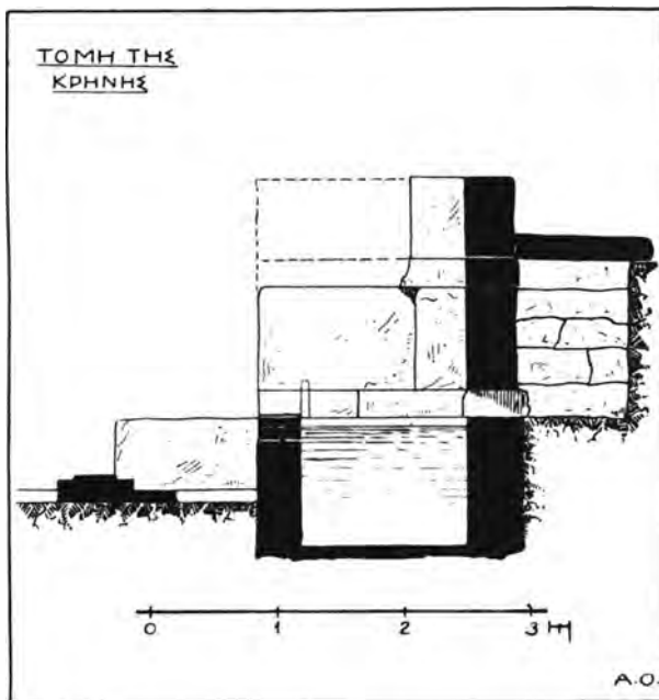
Εἰκ. 3. Τομὴ κατακόρυφος τῆς κρήνης.
