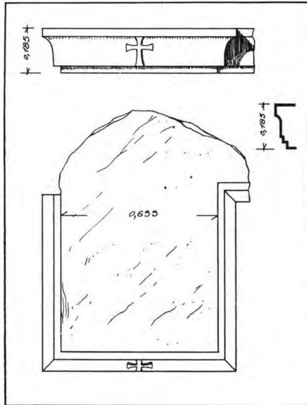
Εἰκ. 11. Κάτοψις καὶ πρόσοψις ἐπικράνου παραστάδος.
