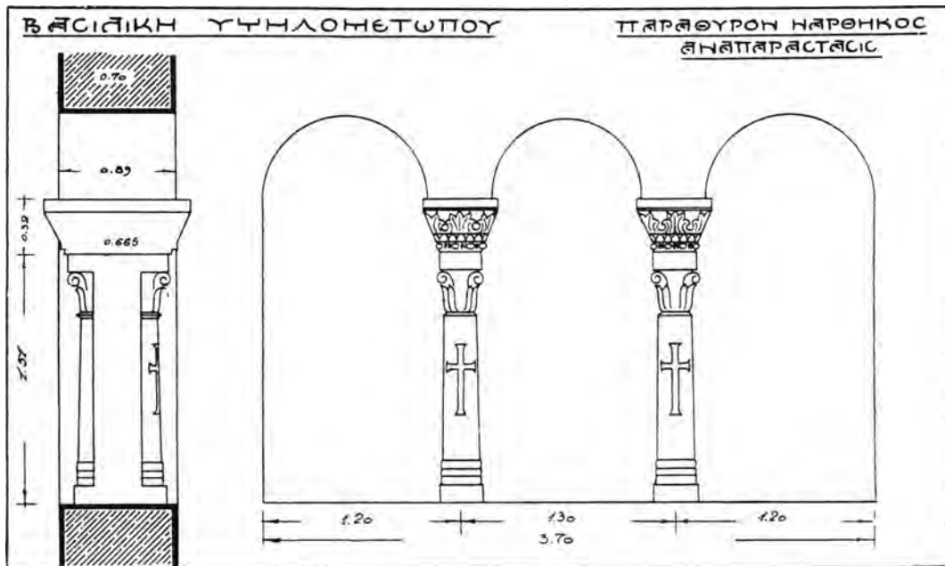
Εἰκ. 5. Ἀναπαράστασις καὶ τομὴ τοῦ παραθύρου τοῦ νάρθηκος.
