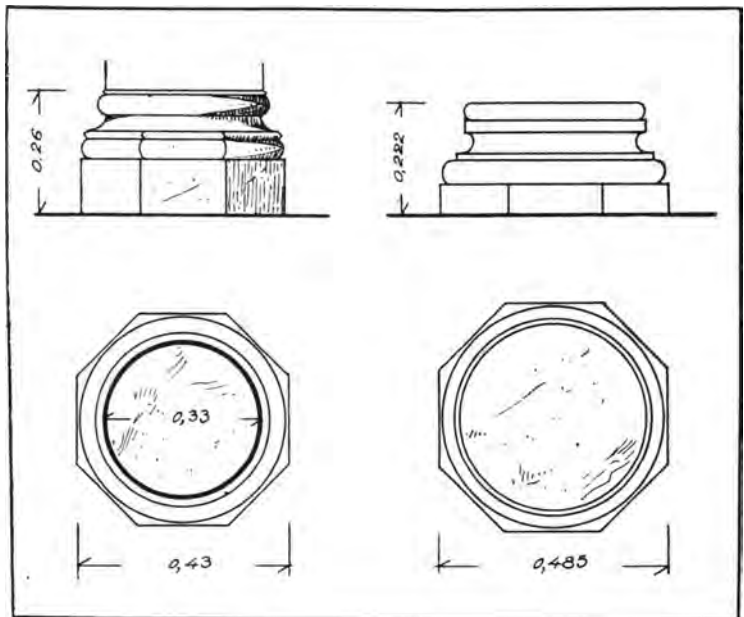
Εἰκ. 14. Βάσεις κίωνων ἄνω ὁρόφου.
