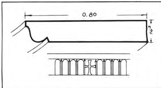
Εἰκ. 12. Καμπύλον γεῖσον (κοσμήτης).
