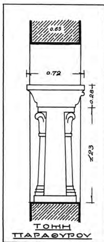
Εἰκ. 23. Τομή παραθύρου.
