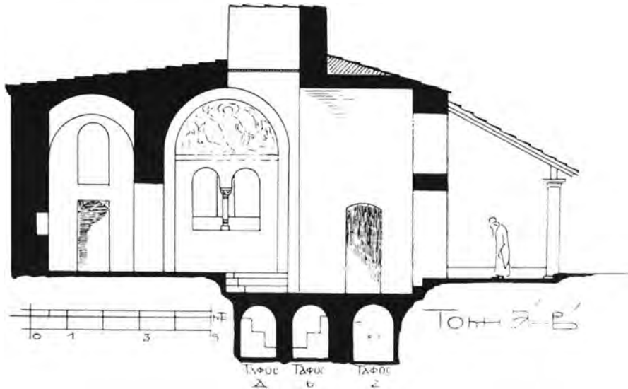
Εἰκ. 3. Τομή κατὰ πλάτος.
