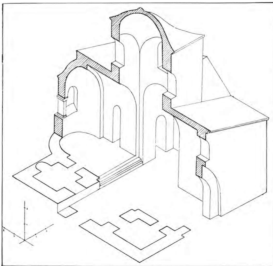
Εἰκ. 7. Τομὴ ἰσομετρικὴ τοῦ μνημείου συμπεπληρωμένον.
