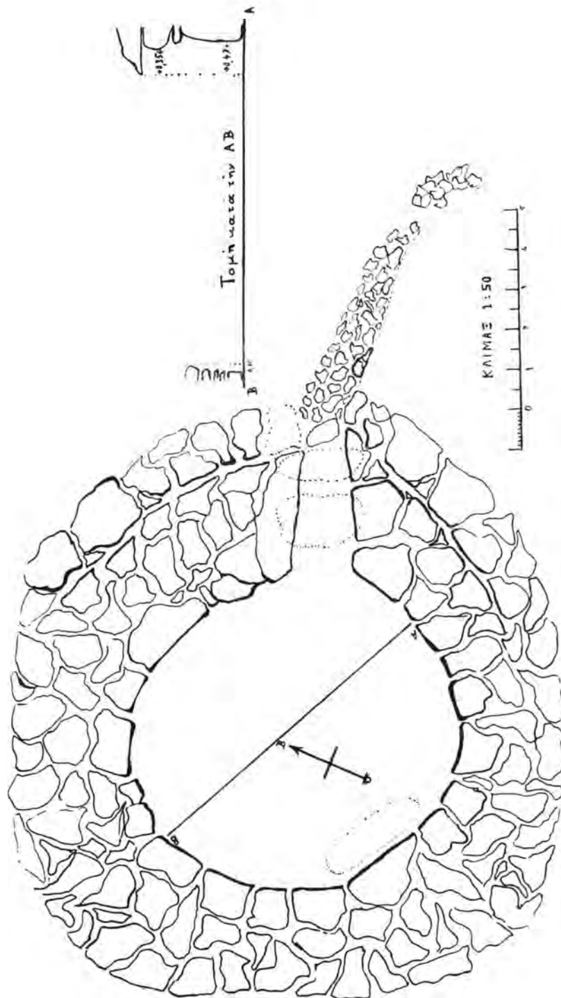
Εἰκὼν 2. Σχέδιον τοῦ τάφου.
