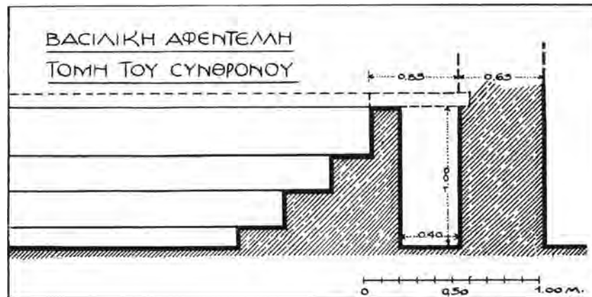
Εἰκ. 50. Τομή τοῦ συνθρόνου.
