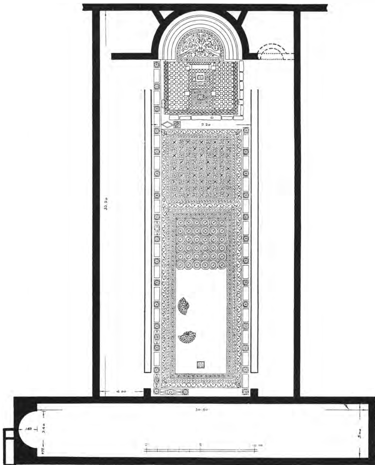
Εἰκ. 46. Κάτοψις τῆς βασιλικῆς Ἀφεντέλλη.
