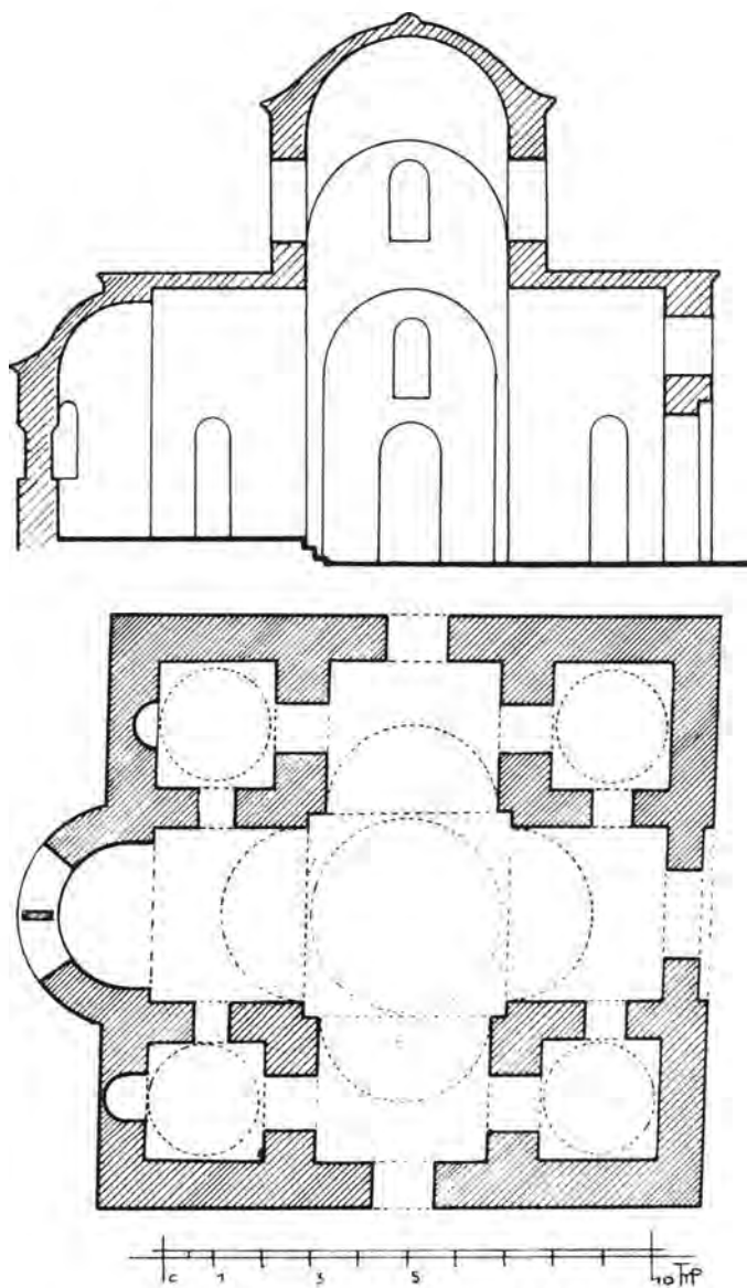
Εἰκ. 4. Κάτοψις καὶ τομὴ συμπεπληρωμέναι.
