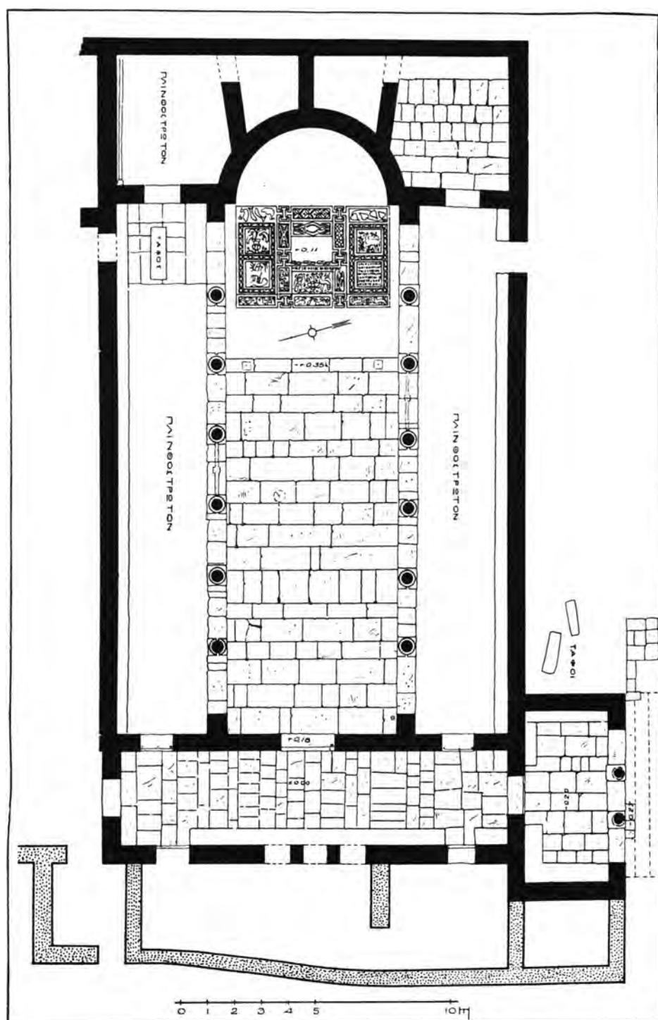
Εἰκ. 1. Κάτοψις τῆς βασιλικῆς Ὑψηλομετώπου.
