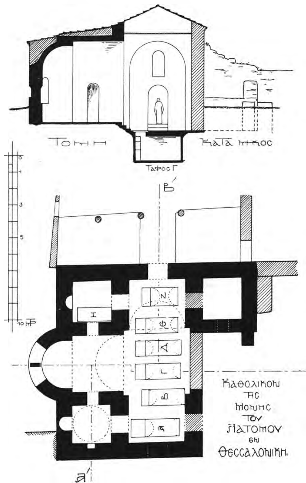
Είκ. 2. Κάτοψις καὶ τομή κατὰ μῆκος τοῦ μνημείου ἐν τῇ νῦν αὐτοῦ καταστάσει.
