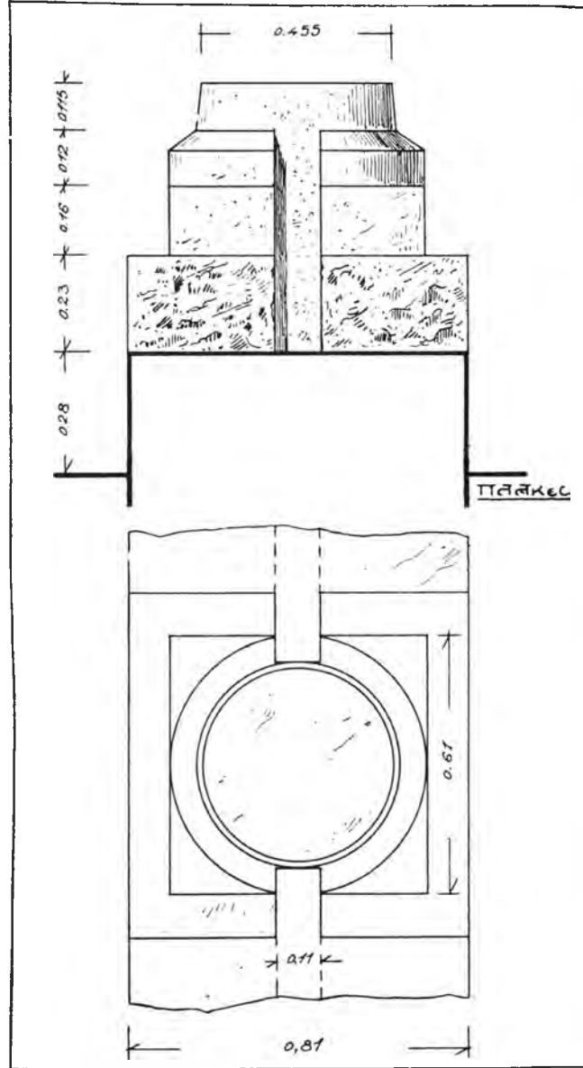
Εἰκ. 7. Κάτοψις καὶ πλαγία ὄψις τῶν βάσεων τῶν κιόνων.
