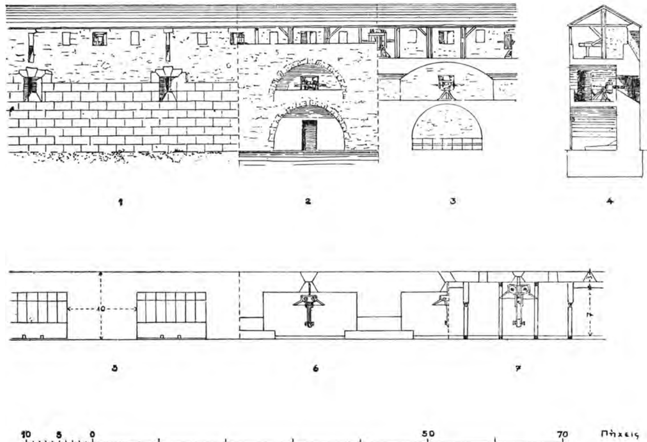
Σχεδ. 3. Ἀναπαράστασις μεσοπυργίου τοῦ τείχους τῆς Ρόδου κατὰ Φίλωνα (Schramm). (1. Ἐξωτερικὴ ὄψις, 2. Ἐσωτερικὴ ὄψις, 3. Κατὰ μῆκος τομή, 4. Ἐγκαρσία τομή, 5. Κάτωγλις ἰσογείου, 6. Κάτωγλις 1ου ὀρόφου, 7. Κάτωγλις 2ου ὀρόφου)
