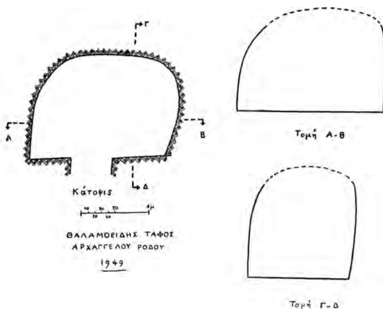
Σχεδ. 1. Κάτοψις καὶ τομή θαλαμοειδοῦς τάφου Ἀρχαγγέλου Ρόδου
