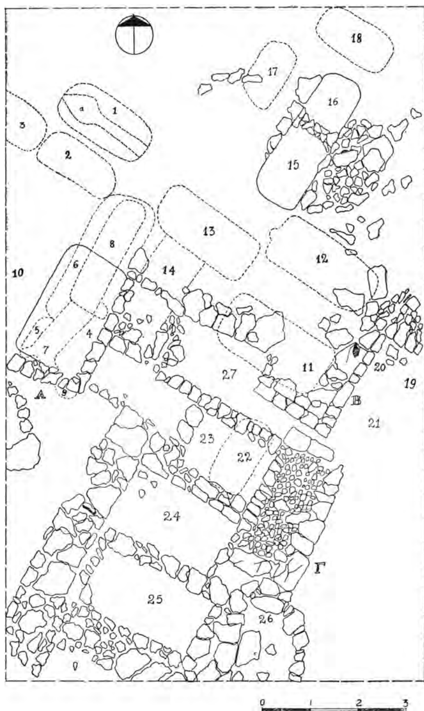
Σχεδ. 1. Βάρη. Κάτοψις ανασκαφής τάφων
