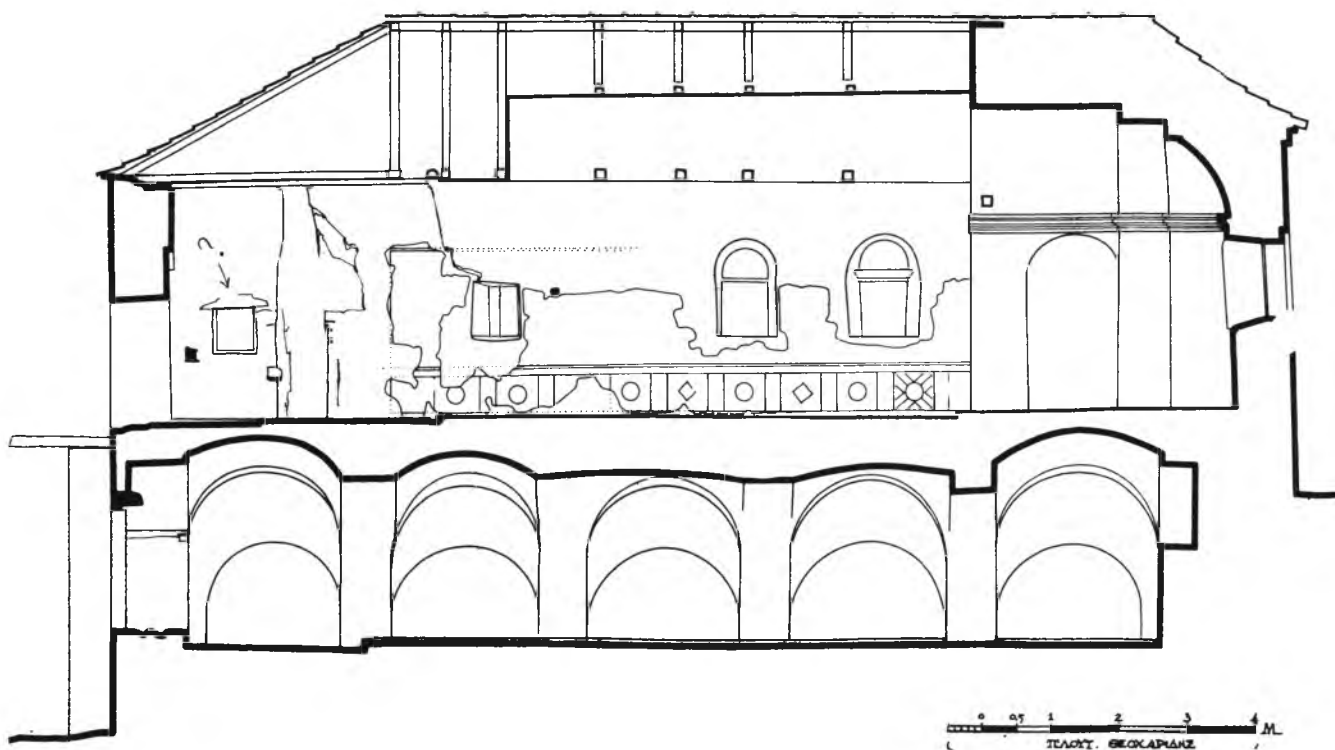
Σχέδ. 2. Άγιον Όρος. Μονή Χελανδαρίου. Κοιμητηριακός ναός του Ευαγγελισμού της Θεοτόκου. Τομή.
