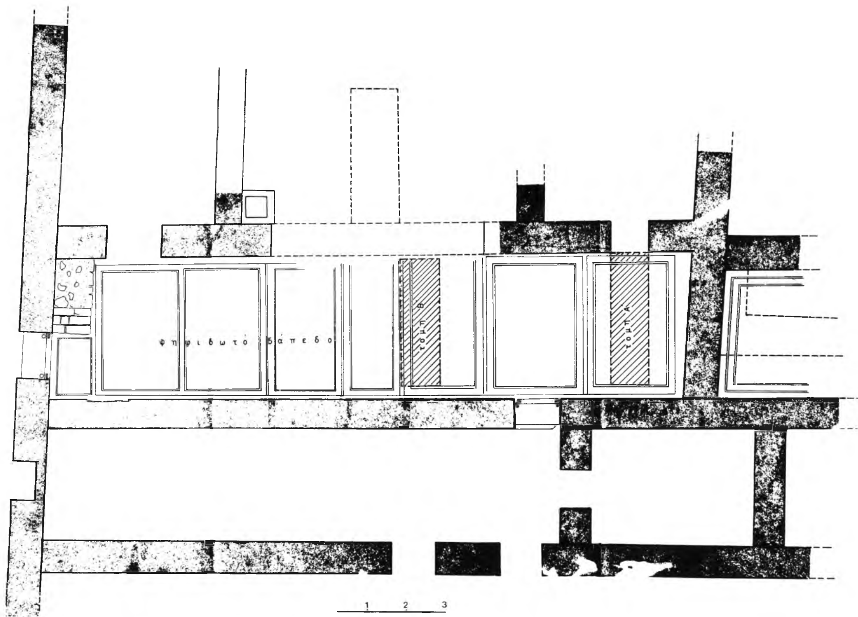
Σχέδ. 2. Ποδοχώρι Παγγαίου. Παλαιοχριστιανική βασιλική. Θέση τομών.
