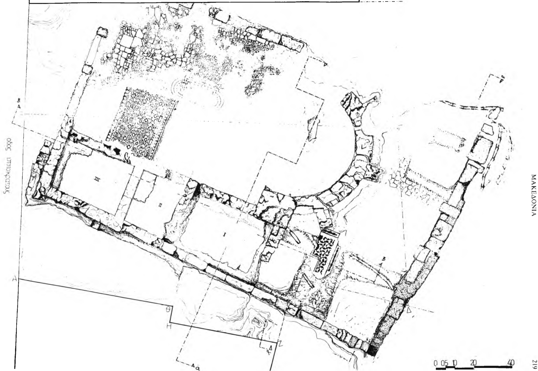
Σχέδ. 1. Βέροια. Οδός Ιπποκράτους και Προφήτου Ηλίου (Ο.Τ. 80). Κάτοψη υστερορωμαϊκής οδού και των οικημάτων στις δύο πλευρές της.
