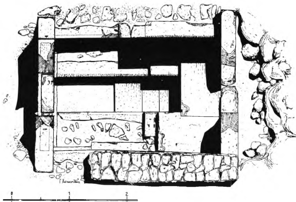
Σχέδ. 1. Πυθαγόρειο Σάμου. Θέση Προφήτης Ηλίας. Κάτοψη του ταφικού μνημείου.
