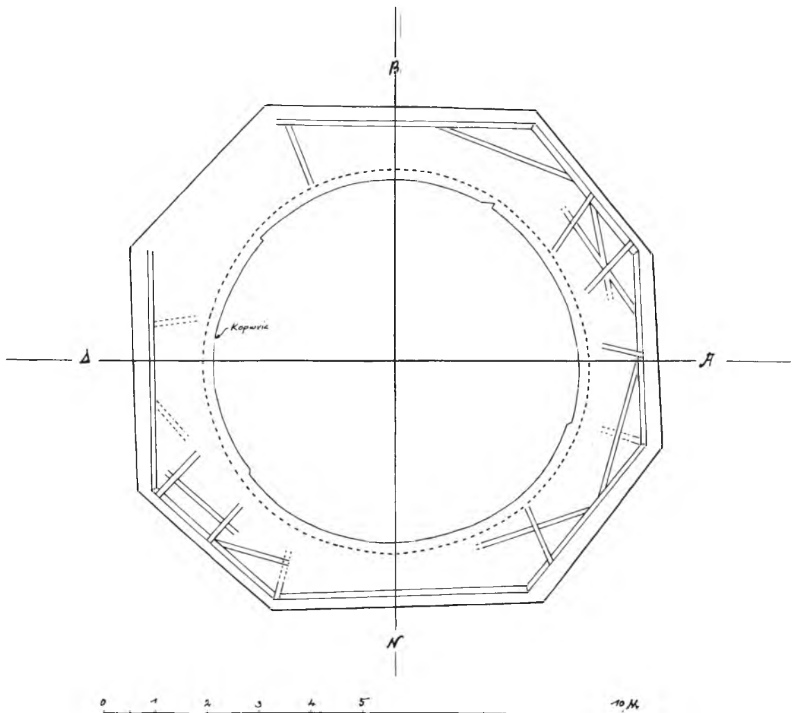
Σχέδ. 4. Φέροι. Παναγία η Κοσμοσώτειρα. Ξυλοδεσιά στην οκτάγωνη βάση του τρούλου.
