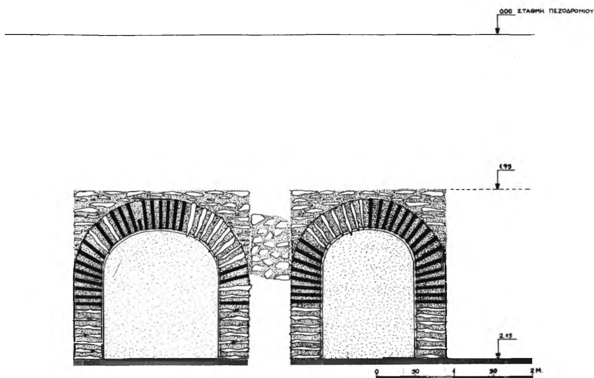
Σχέδ. 3. Θεσσαλονίκη. Οδός Ελευθερίας 13. Τομή Α-Β τάφου.
