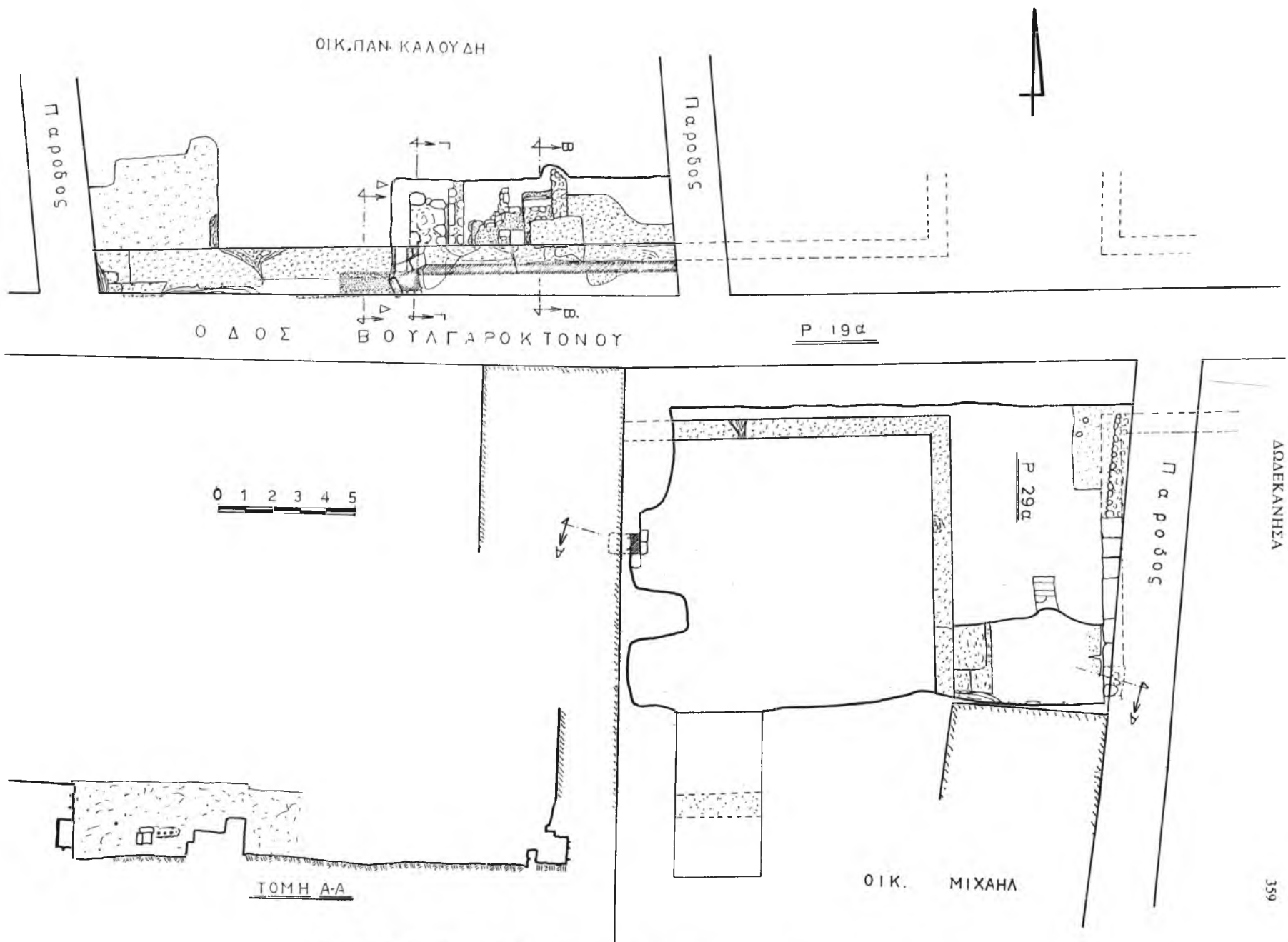
Σχέδ. 8. Ρόδος. Οικόπεδα Μιχαήλ και Καλούδη. Κάτοψη της ανασκαφής και τομή Α-Α.
