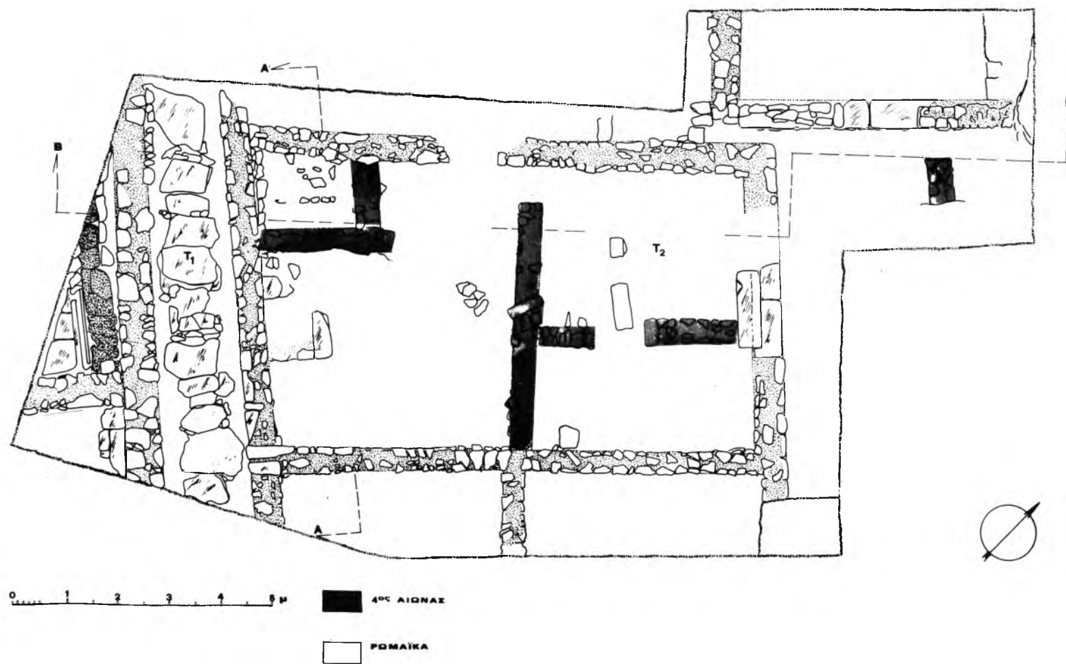
Σχέδ. 4. Θάσος, Λιμένας. Οικόπεδο Ι. Μυρώνη. Κάτοψη της ανασκαφής.
