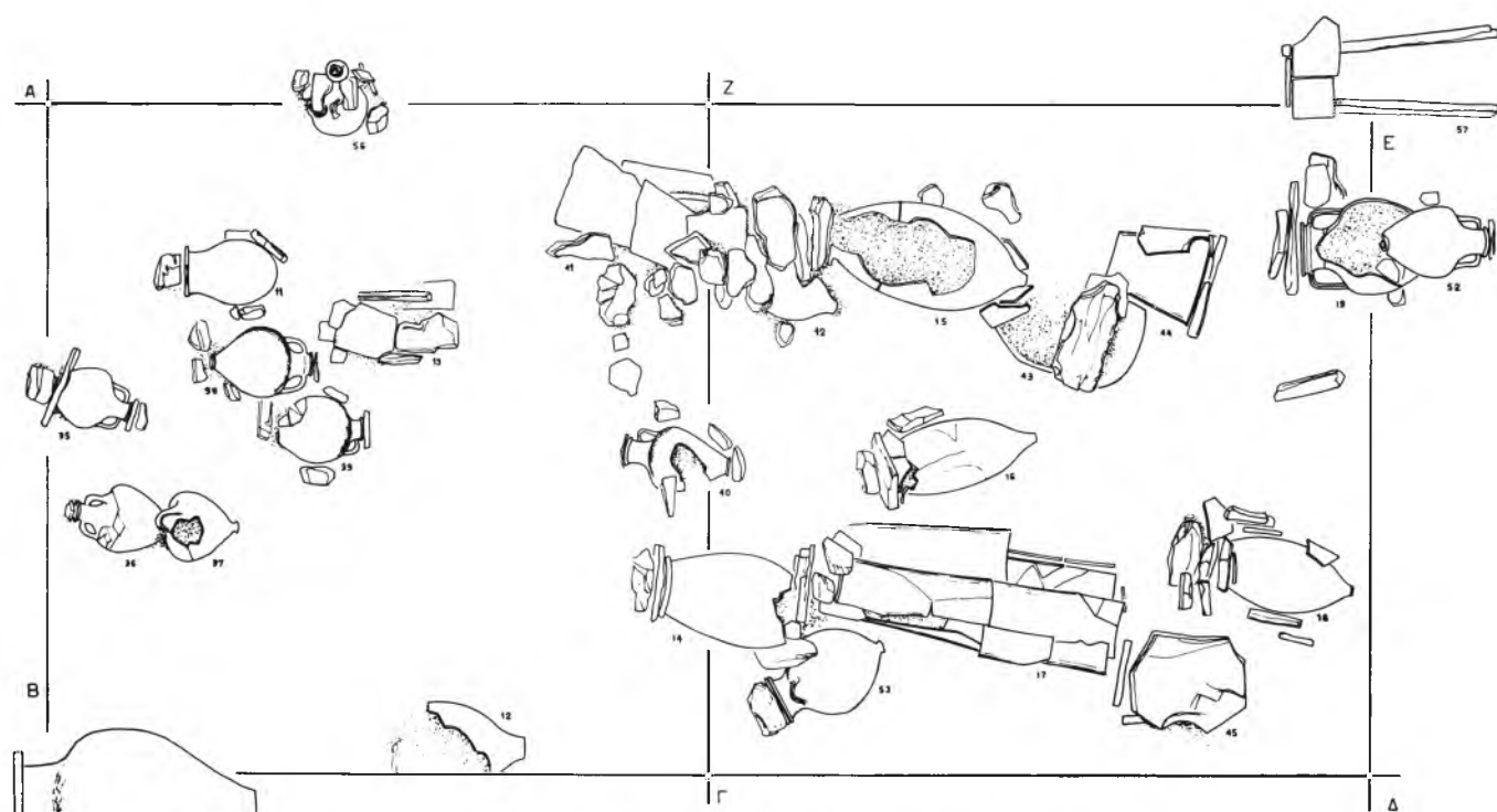
Σχέδ. 6. Χαλκιδική. Νικήτη. Ἅγιος Ιωάννης. Δοκιμαστική τομή 6. Φάση α'.
