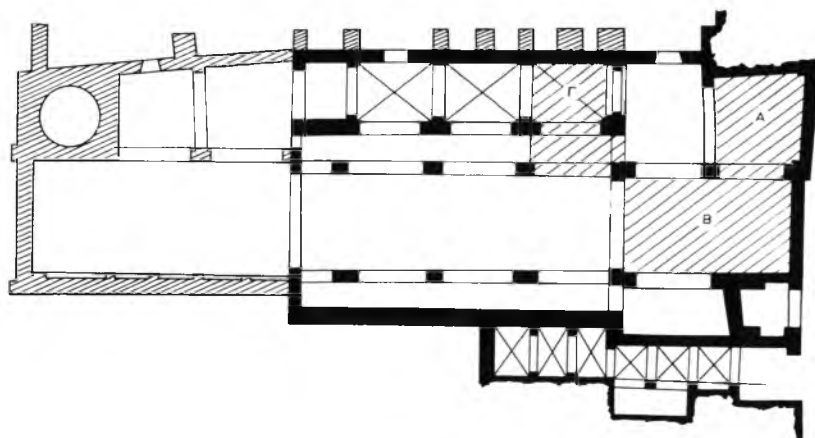
Σχέδ. 3. Αρχαιολογικό Μουσείο Χανίων (ναός Αγίου Φραγκίσκου). Κάτοψη.
