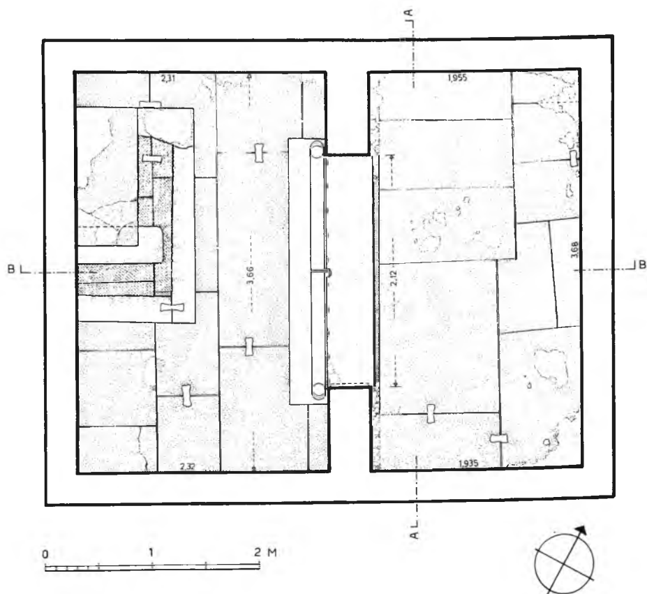
Σχέδ. Ι. Κατερίνη. Κάτοψη Μακεδονικού τάφου Α.
