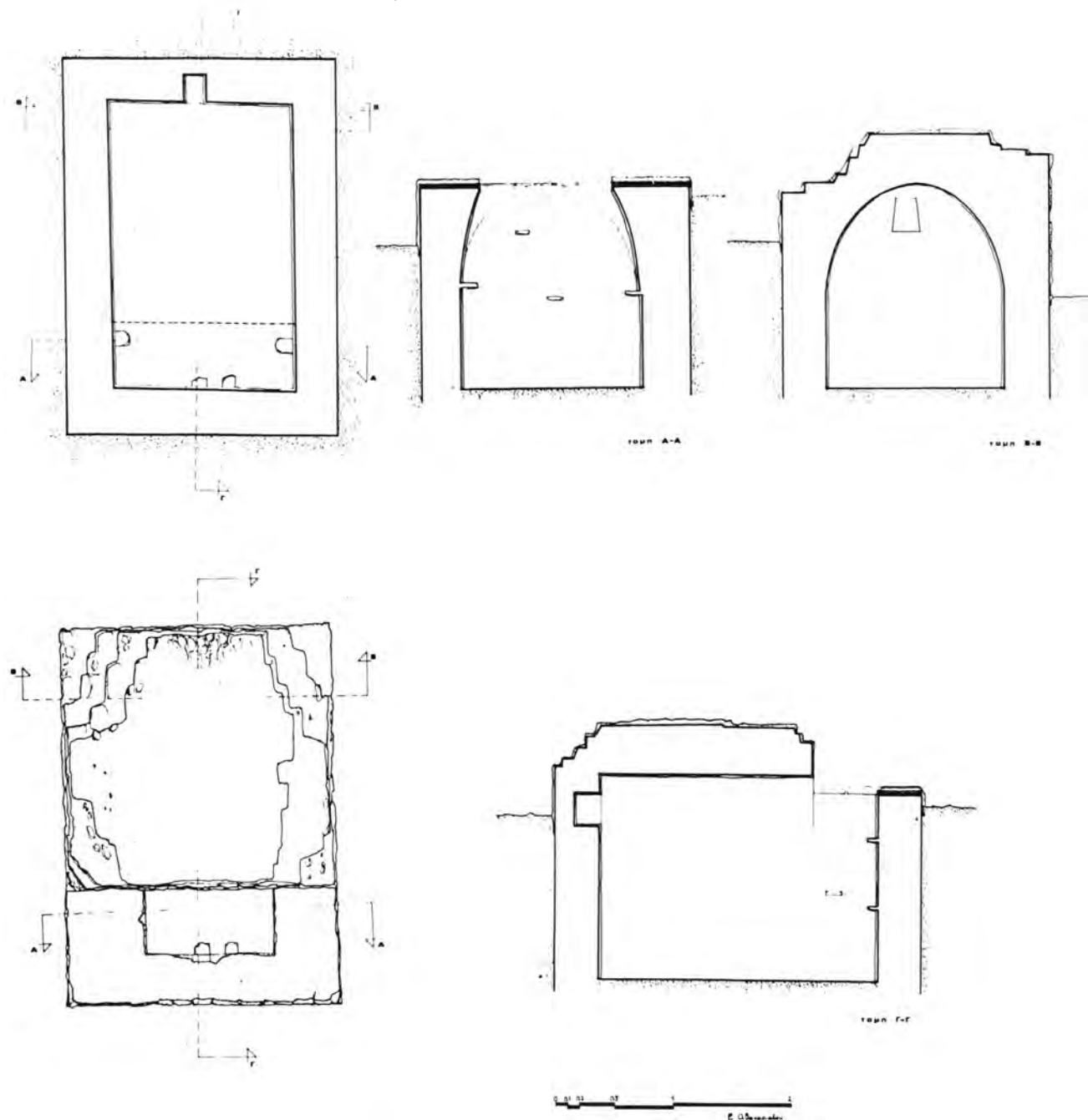
Σχέδ. 9. Πυλαία Θεσσαλονίκης. Οδός Προφήτη Ηλία 36. Κατόψεις και τομές του τάφου.
