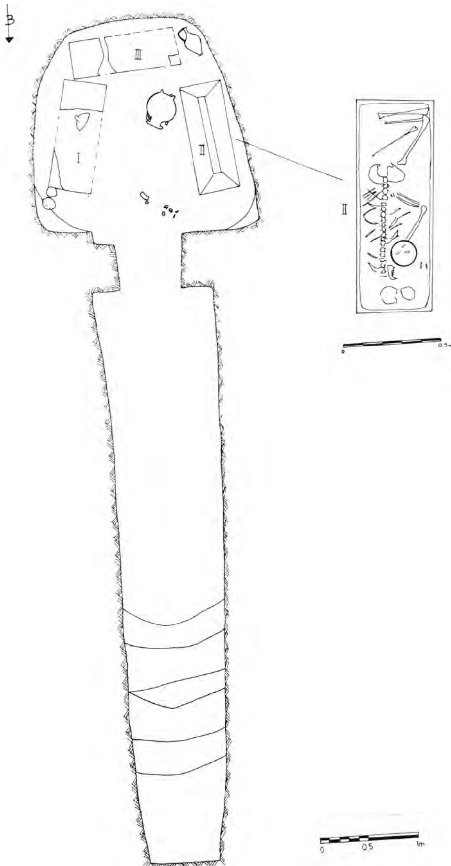
Σχέδ. 6. Παγκαλοχώρι Ρεθύμνου. Κάτοψη του ΥΜ ΙΙΙ θαλαμωτού τάφου.
