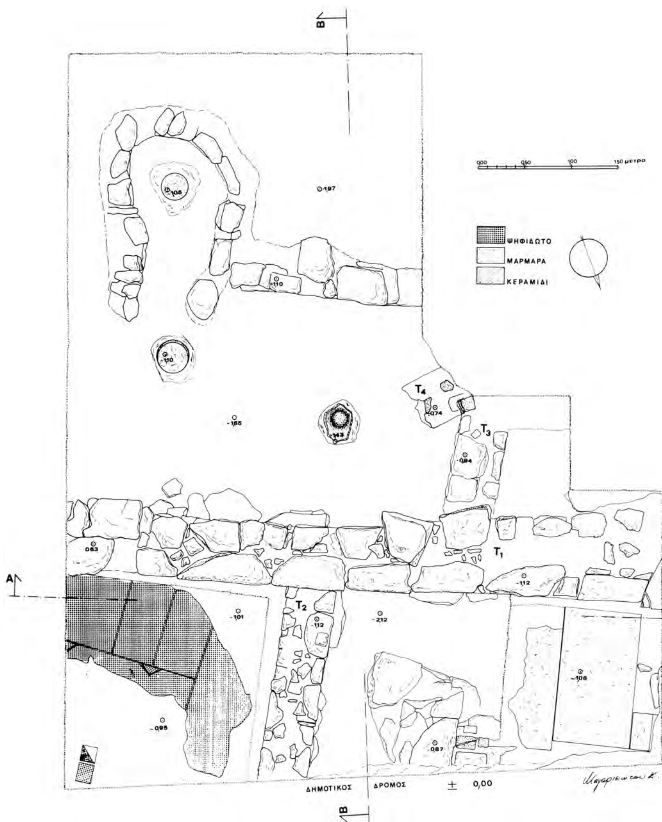
Σχέδ. 1. Λιμένας Θάσου. Οικόπεδο Ι. Καζάρα. Κάτοψη της ανασκαφής.
