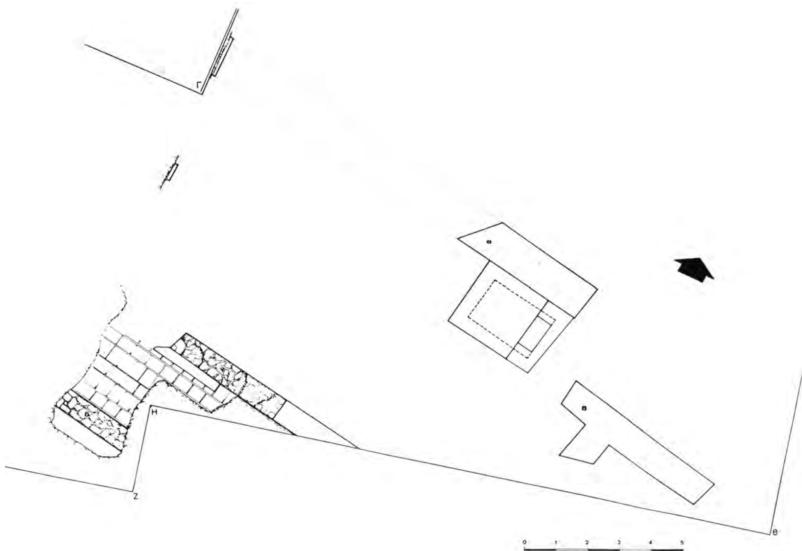
Σχέδ. 8. Πυλαία Θεσσαλονίκης. Οδός Προφήτη Ηλία 36. Κάτοψη της ανασκαφής.
