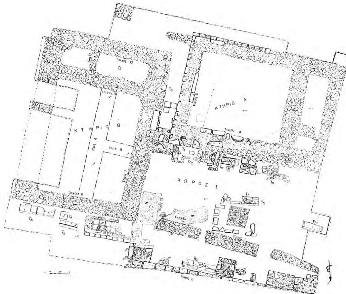
Σχέδ. 2. Κέρκυρα. Ανεμόμυλος. Οικόπεδο Αικ. Σταθοπούλου. Κάτοψη της ανασκαφής.
