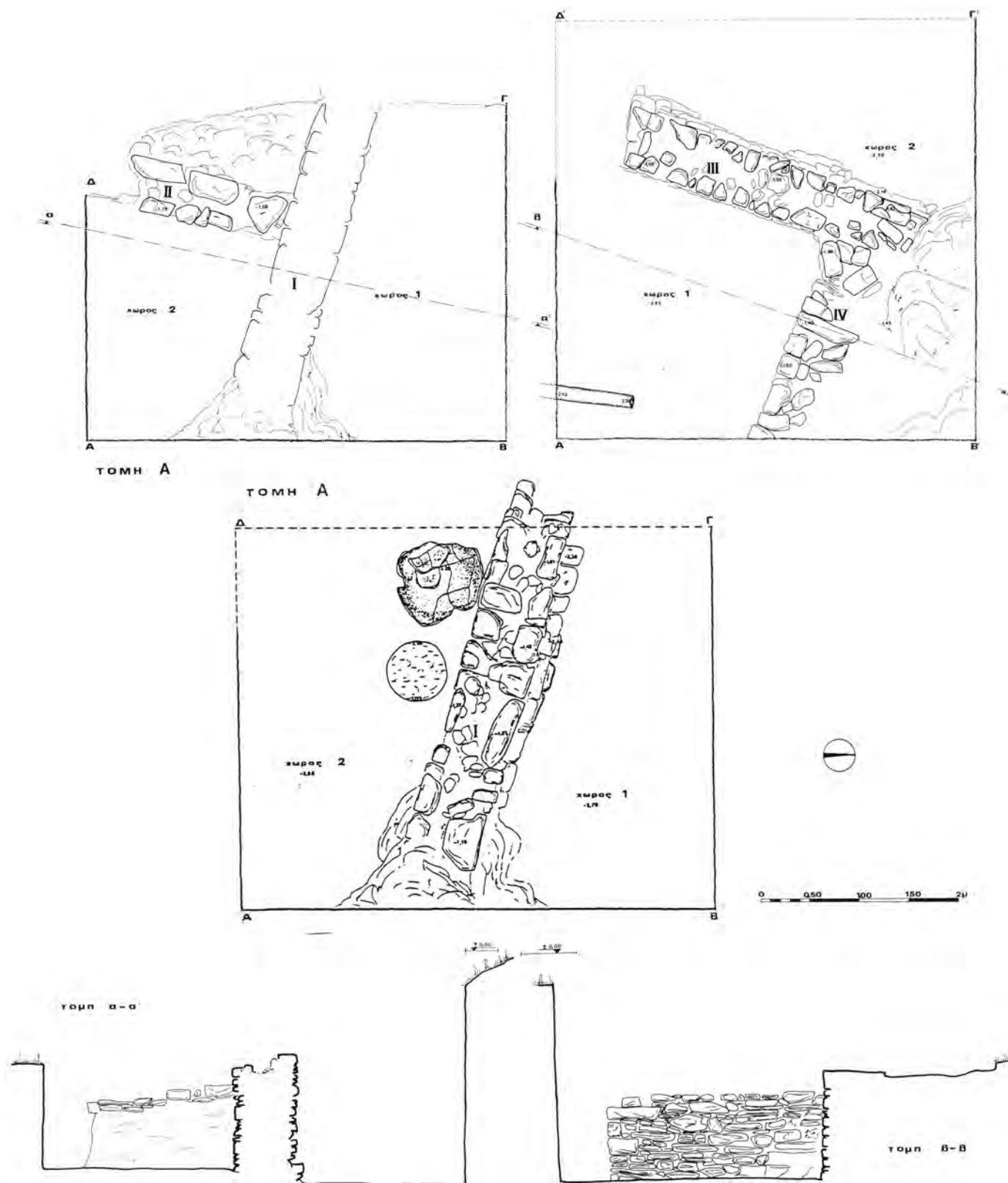
Σχέδ. 5. Θεολόγος Θάσου. Άγιος Ιωάννης Λουκάς. Κτήμα Γρ. Παπαδόπουλου. Κατόψεις και τομές αα' και ββ' της ανασκαφής.
