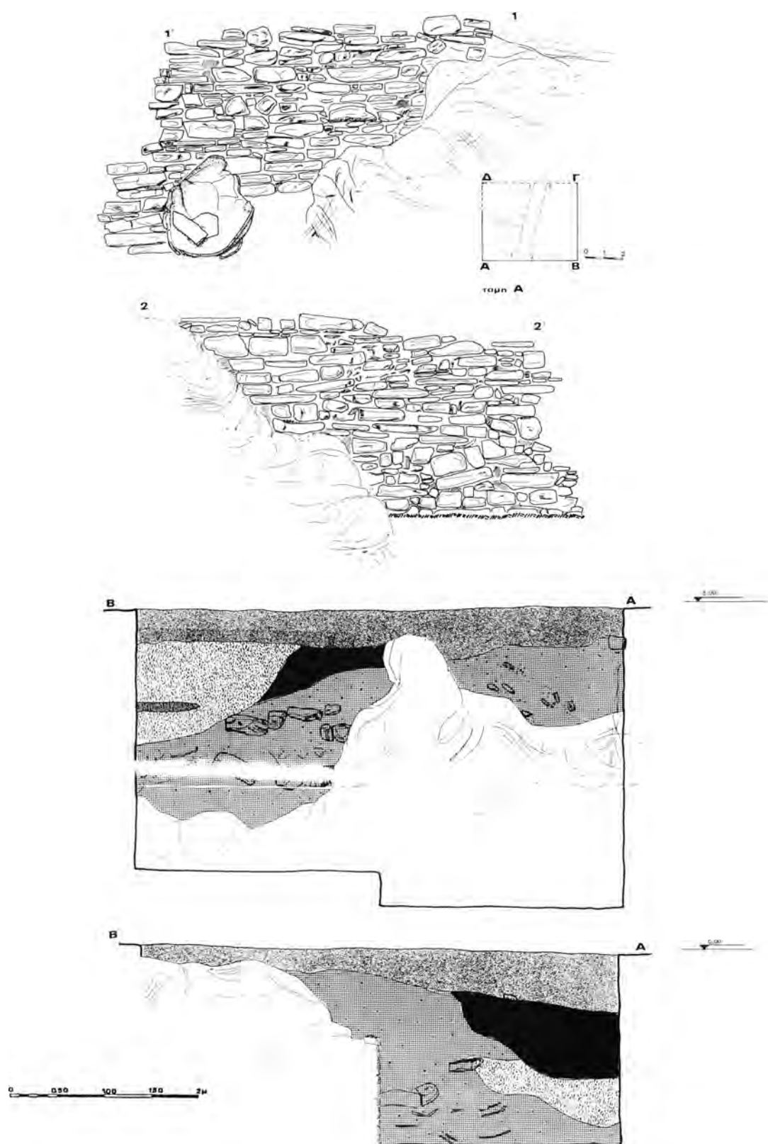
Σχέδ. 6. Θεολόγος Θάσου. Άγιος Ιωάννης Λουκάς. Κτήμα Γρ. Παπαδόπουλου. Όψεις του τοίχου Ι και στρωματογραφίες της ανασκαφής.
