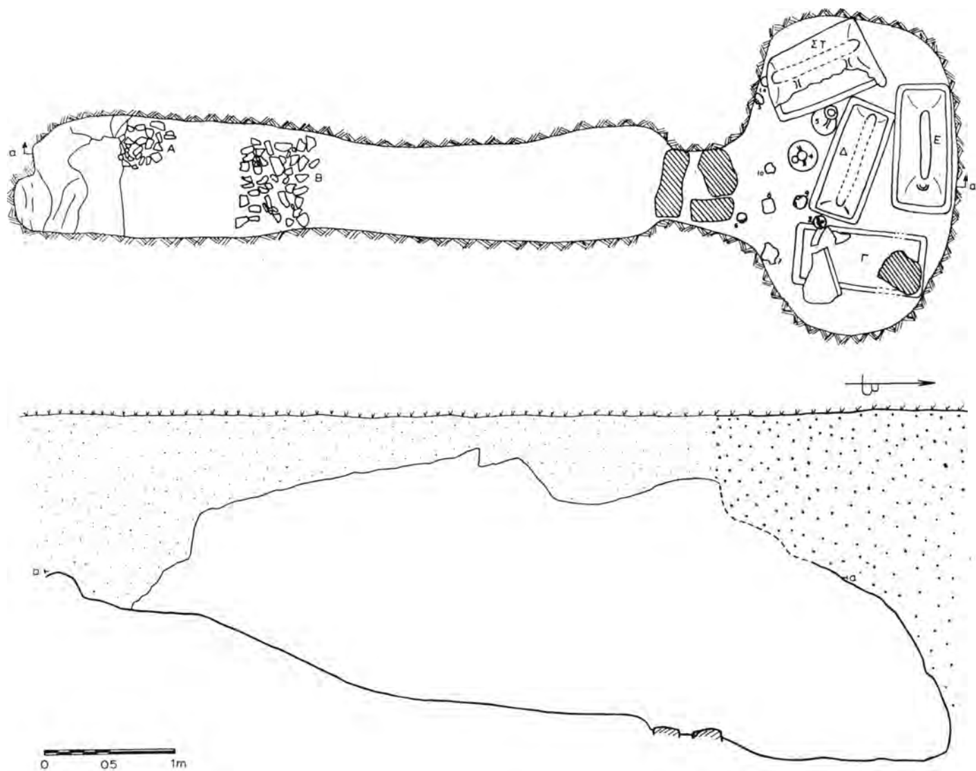
Σχέδ. 5. Αγγελιανά Μυλοποτάμου. Κάτοψη και τομή αα' του ΥΜ θαλαμωτού τάφου.
