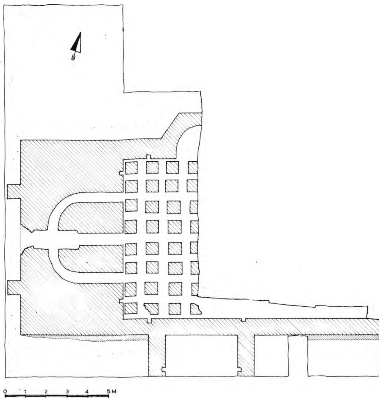
Σχέδ. 2. Ιωάννινα. Βυζαντινό λουτρό. Κάτοψη στη στάθμη των υποκαύστων.
