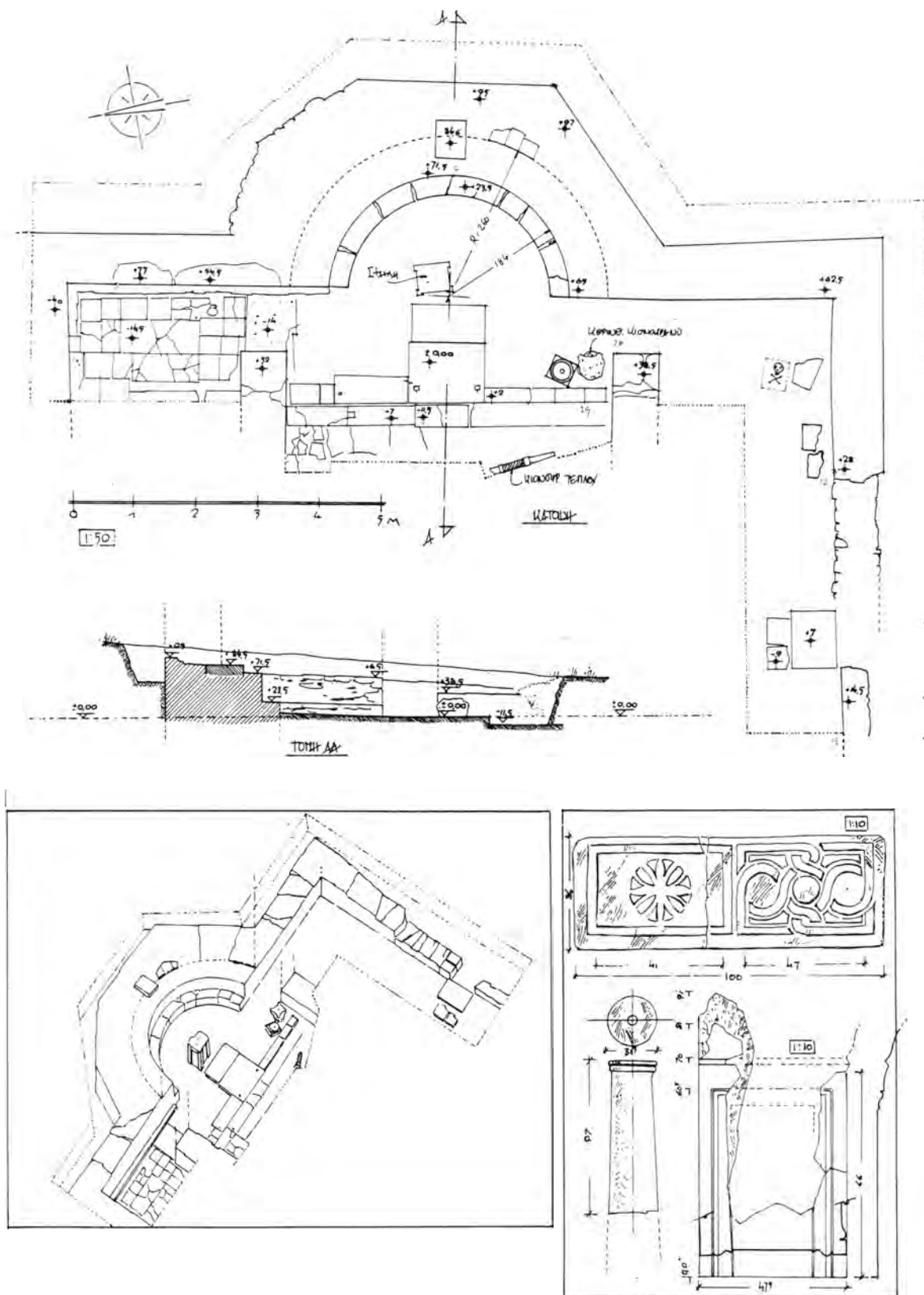
Σχέδ. 10. Κίτρος Πιερίας. Κάτοψη, τομή, αξονομετρική αποτύπωση της αψίδας παλαιοχριστιανικής βασιλικής και λεπτομέρειες αρχιτεκτονικών μελών.
