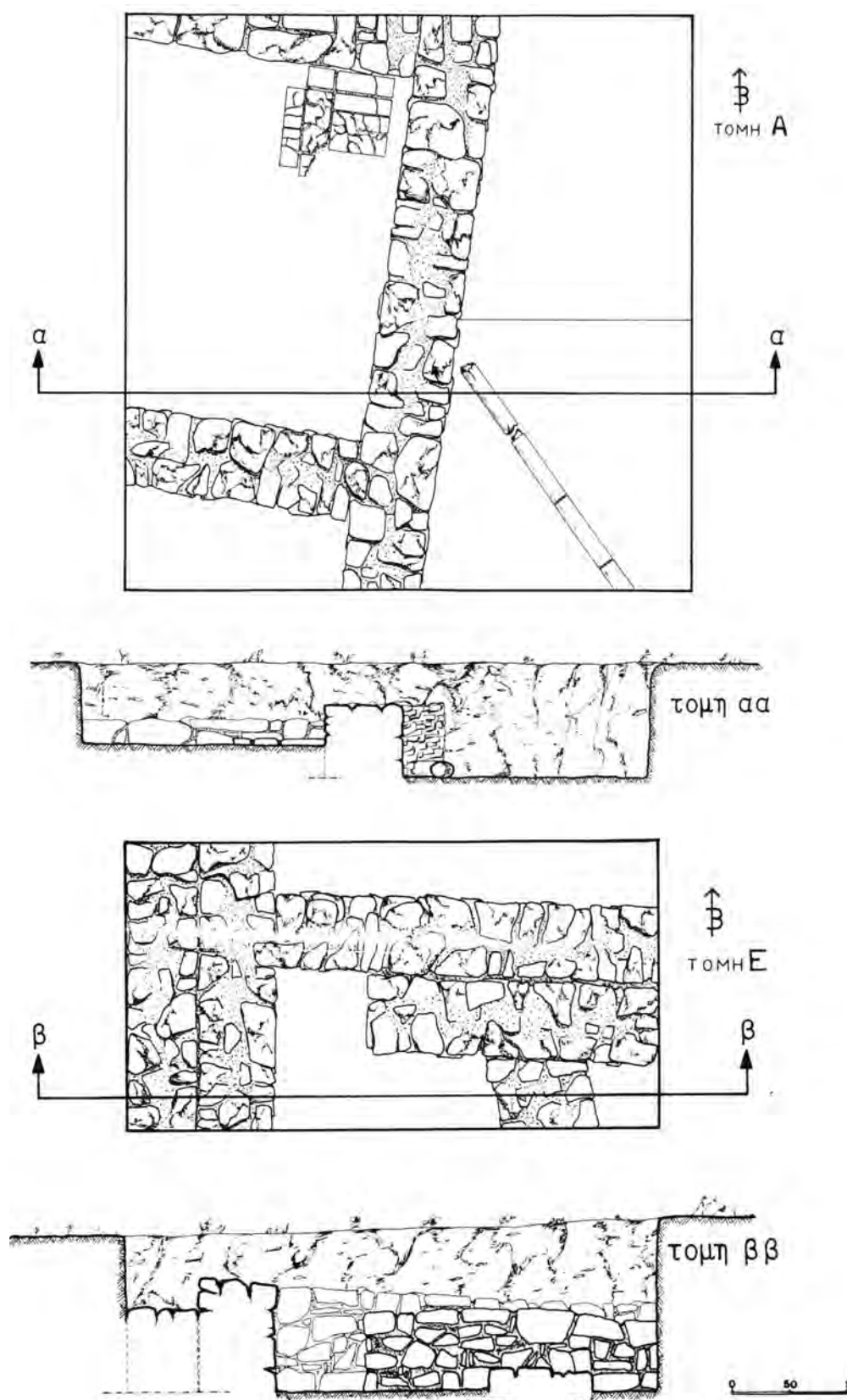
Σχέδ. 3. Καλαμωτό Ζαγκλιβερίου. Κατόψεις των τομών Α, Ε και οι τομές αα και ββ.
