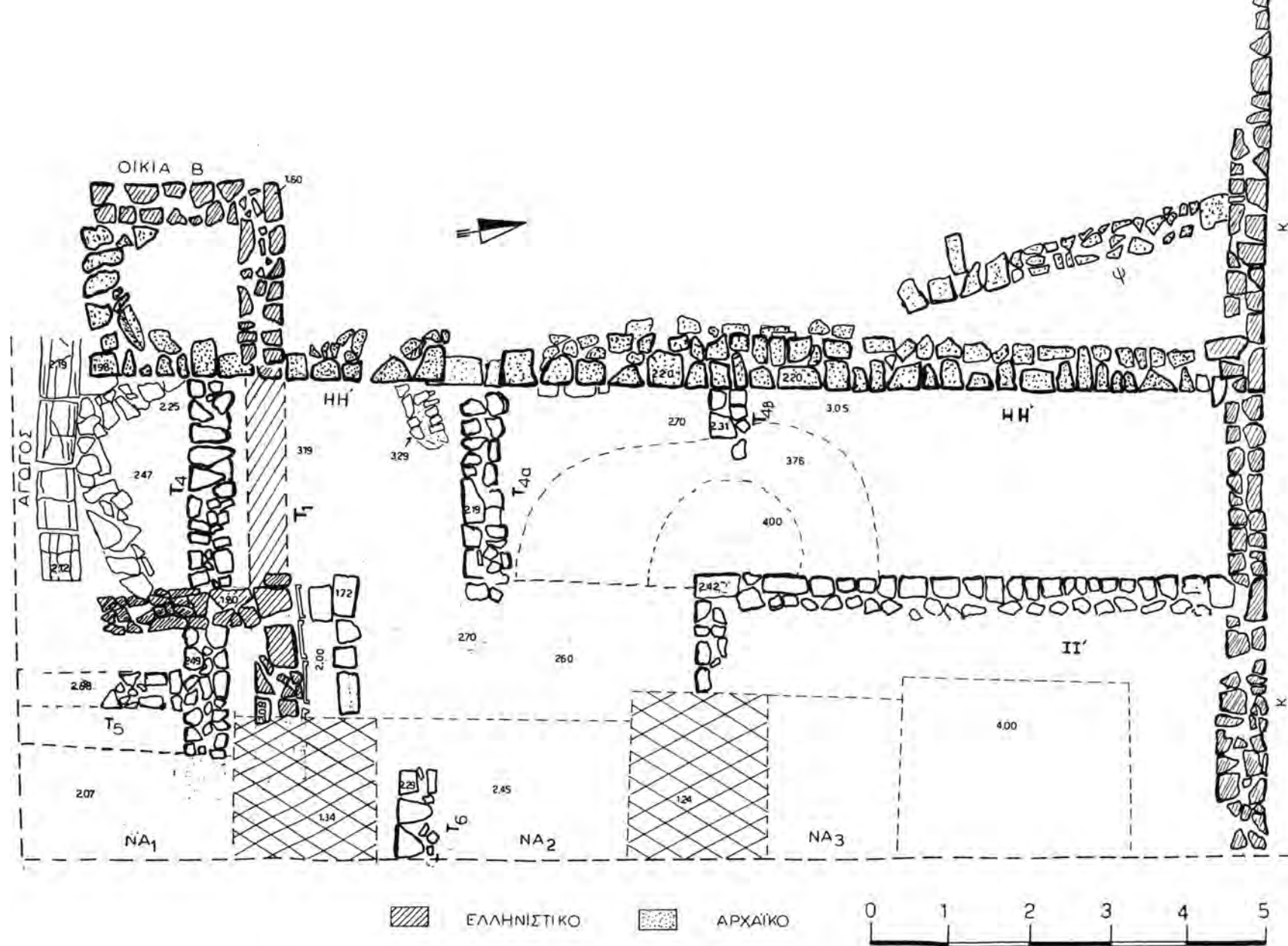
Σχέδ. 3. Κέρκυρα. Ανασκαφή Ευελπίδη. Κάτοψη της ανασκαφής.
