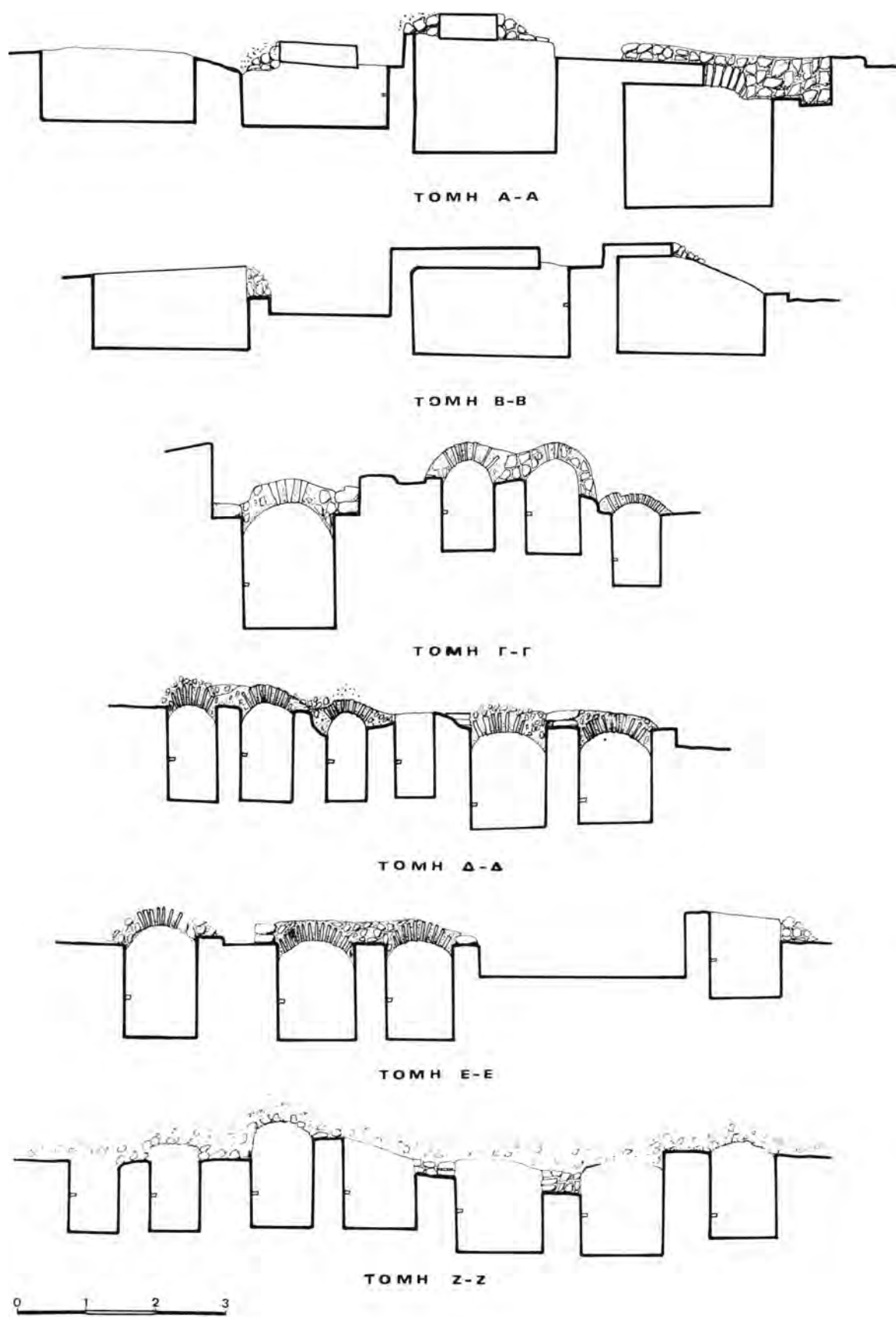
Σχέδ. 2. Θεσσαλονίκη. Λεωφόρος Καλλιθέας 5. Τομές των τάφων.
