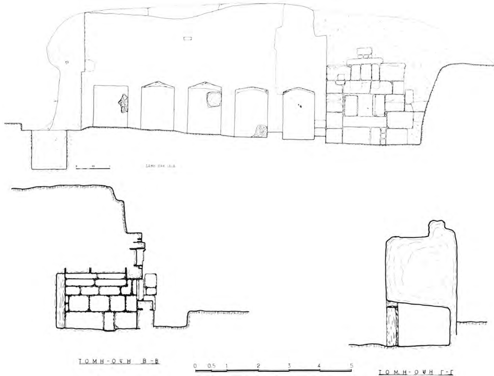
Σχέδ. 3. Ρόδος. Οικόπεδο Κωνστ. Παπασταματίου. Τομές και όψεις της ανασκαφής.
