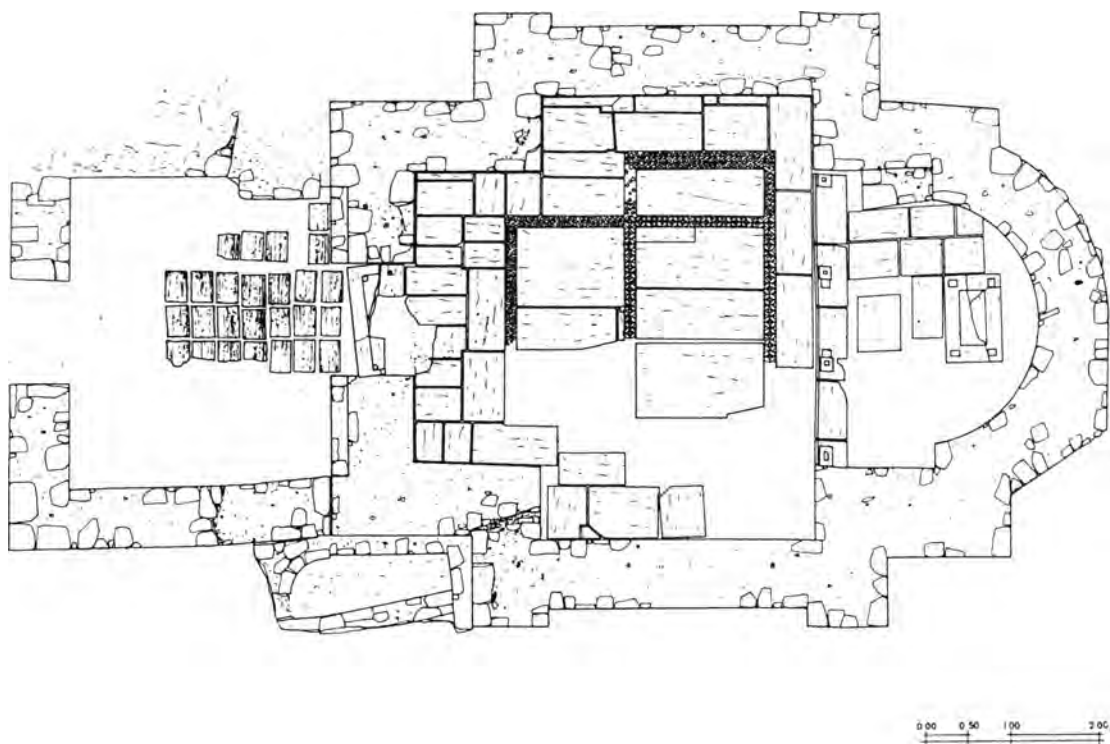
Σχέδ. 2. Κερασιά Ροδόπης. Κάτοψη βυζαντινού ναού.
