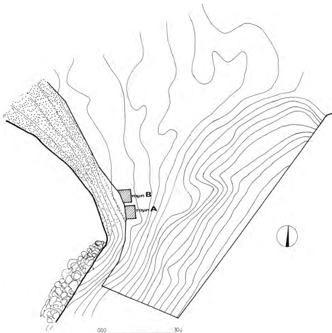
Σχέδ. 4. Θεολόγος Θάσου. Άγιος Ιωάννης Λουκάς. Τοπογραφικό απόσπασμα του κτήματος Γρ. Παπαδόπουλου.
