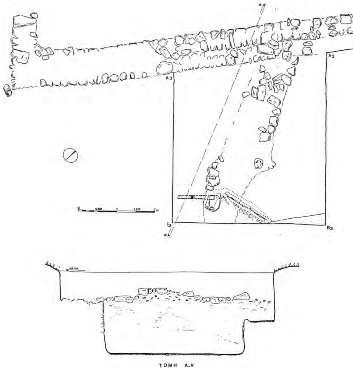
Σχέδ. 8. Βέργη. Κάτοψη ανασκαφικής τομής 3 και τομή ΑΑ'.
