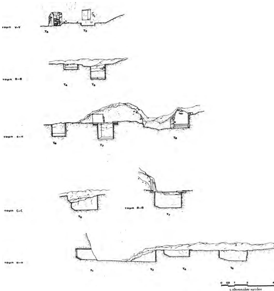
Σχέδ. 7. Θεσσαλονίκη. Οδός Μιχαλά 41. Τομές των τάφων.
