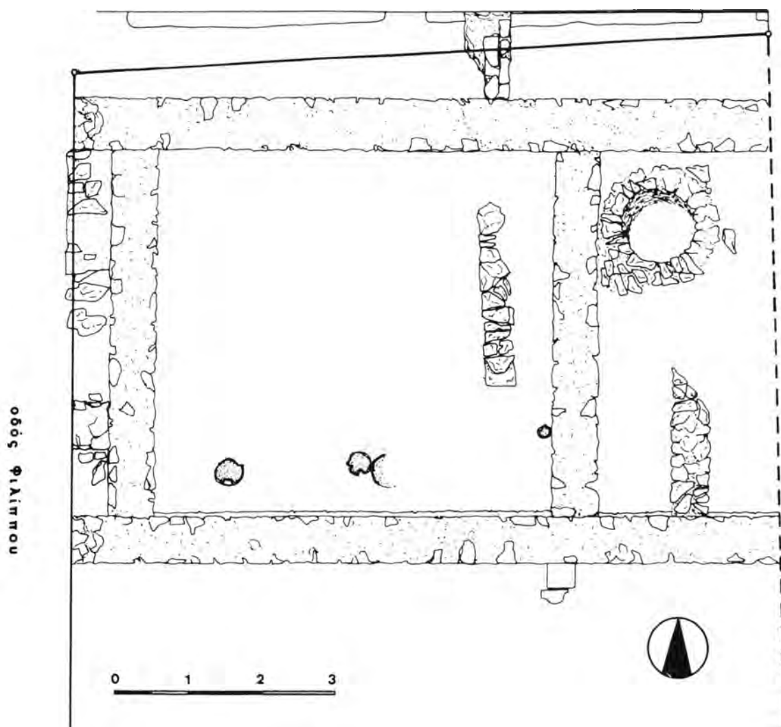
Σχέδ. 2. Θεσσαλονίκη. Οδός Φιλίππου 89. Κάτοψη της ανασκαφής.
